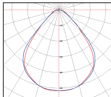
Typische Lichtverteilung
